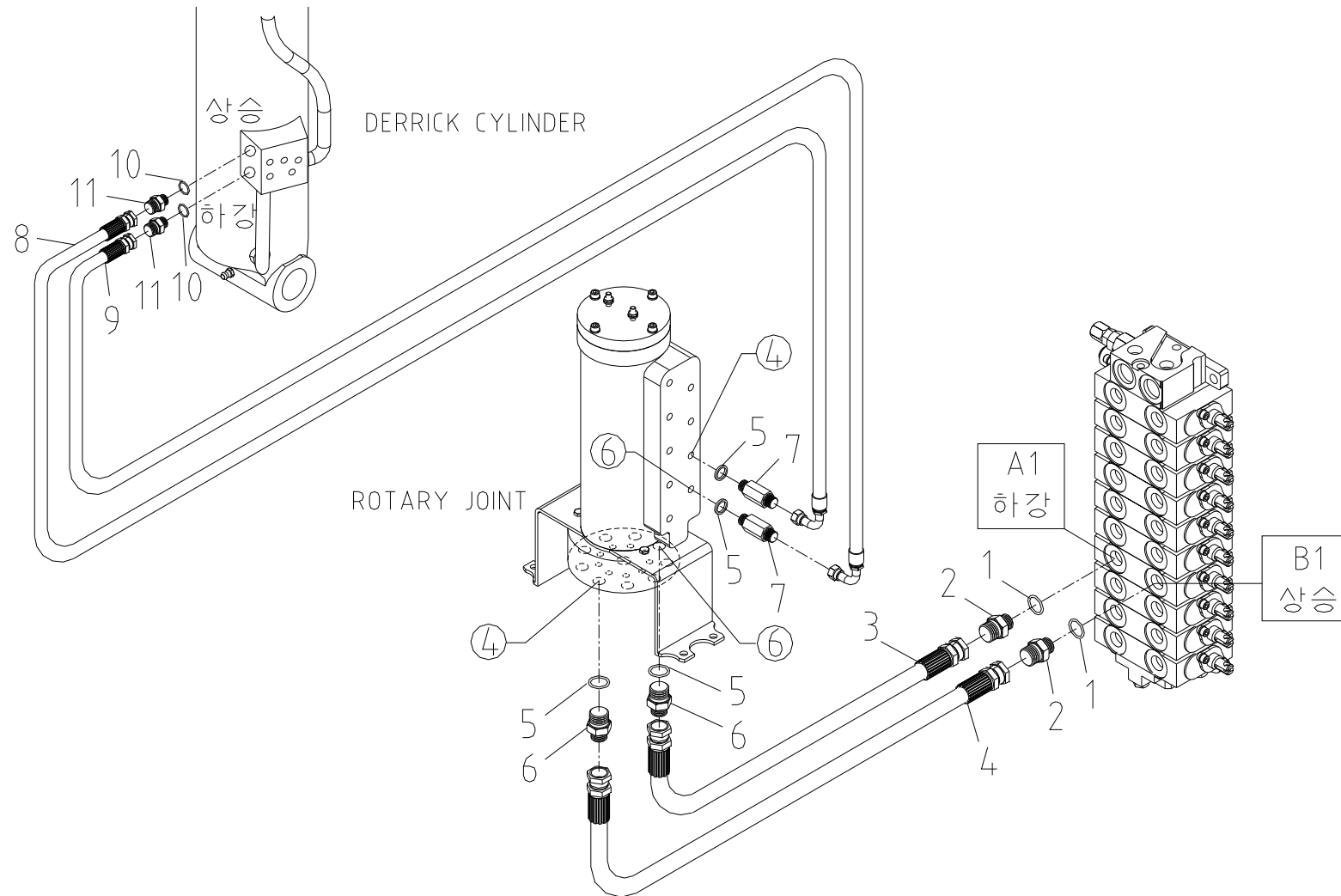
데릭 배관 Fig. 4-2 SAC-2501 DERRICK PIPING
