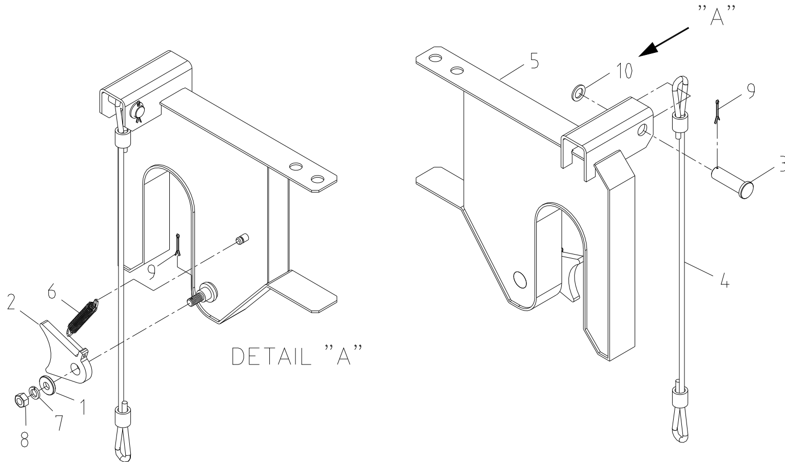
오거 브라켓 조립체 Fig. 1-2 SAC-2501 AUGER BRACKET ASS'Y
