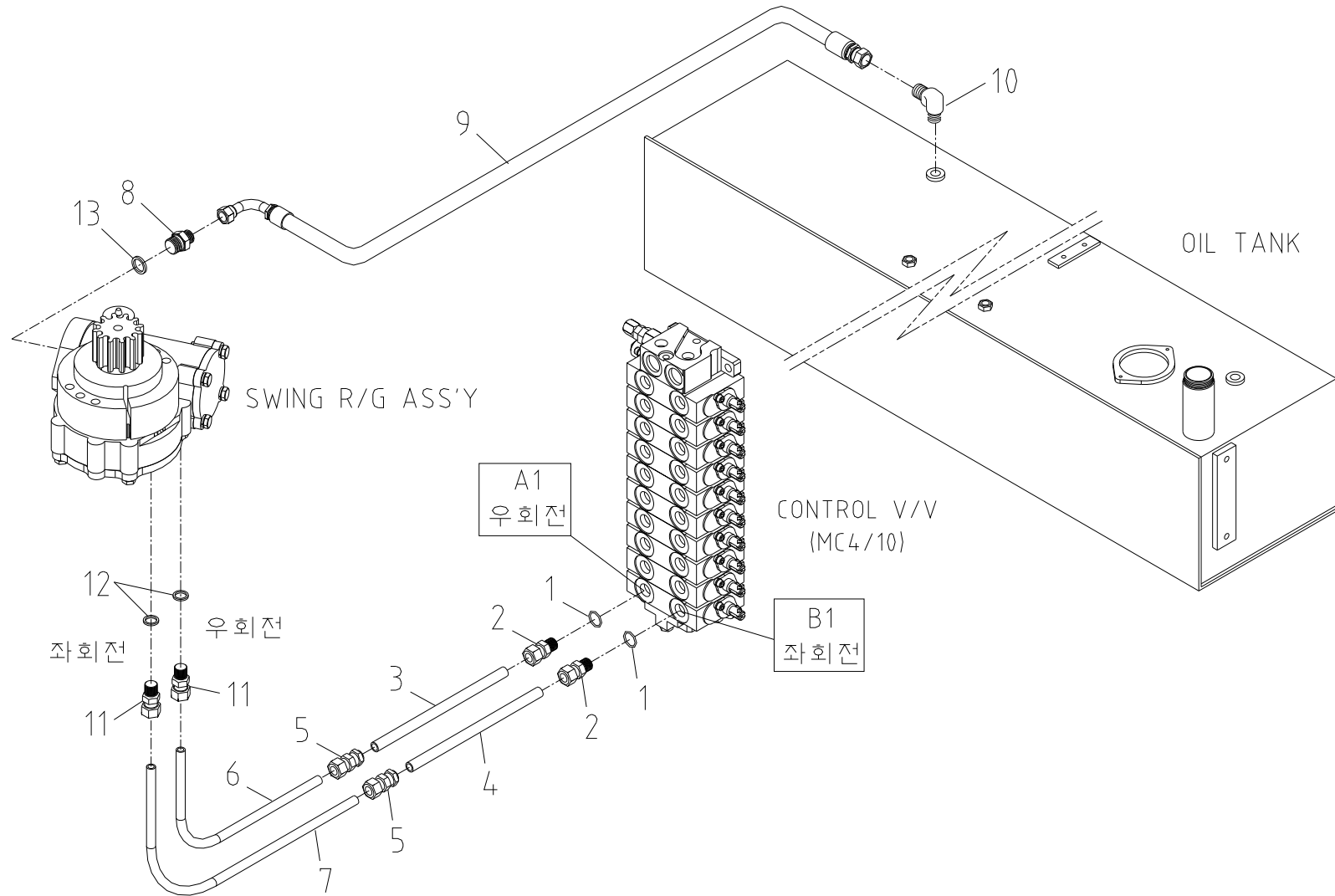
스윙 배관 Fig. 4-5 SAC-2501 SWING PIPING
