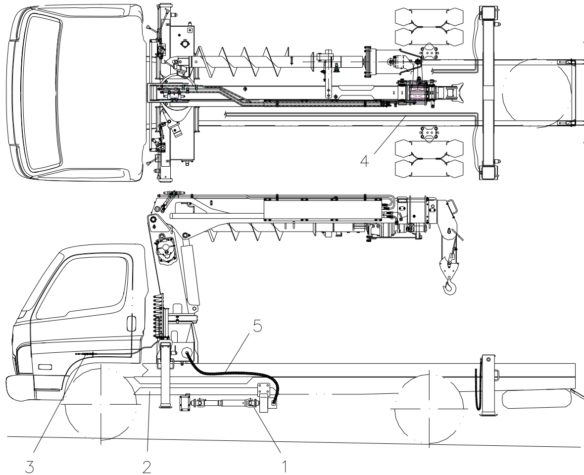
장착 조립체 Fig. 8 SAC-2501 MOUNTING ASS'Y
