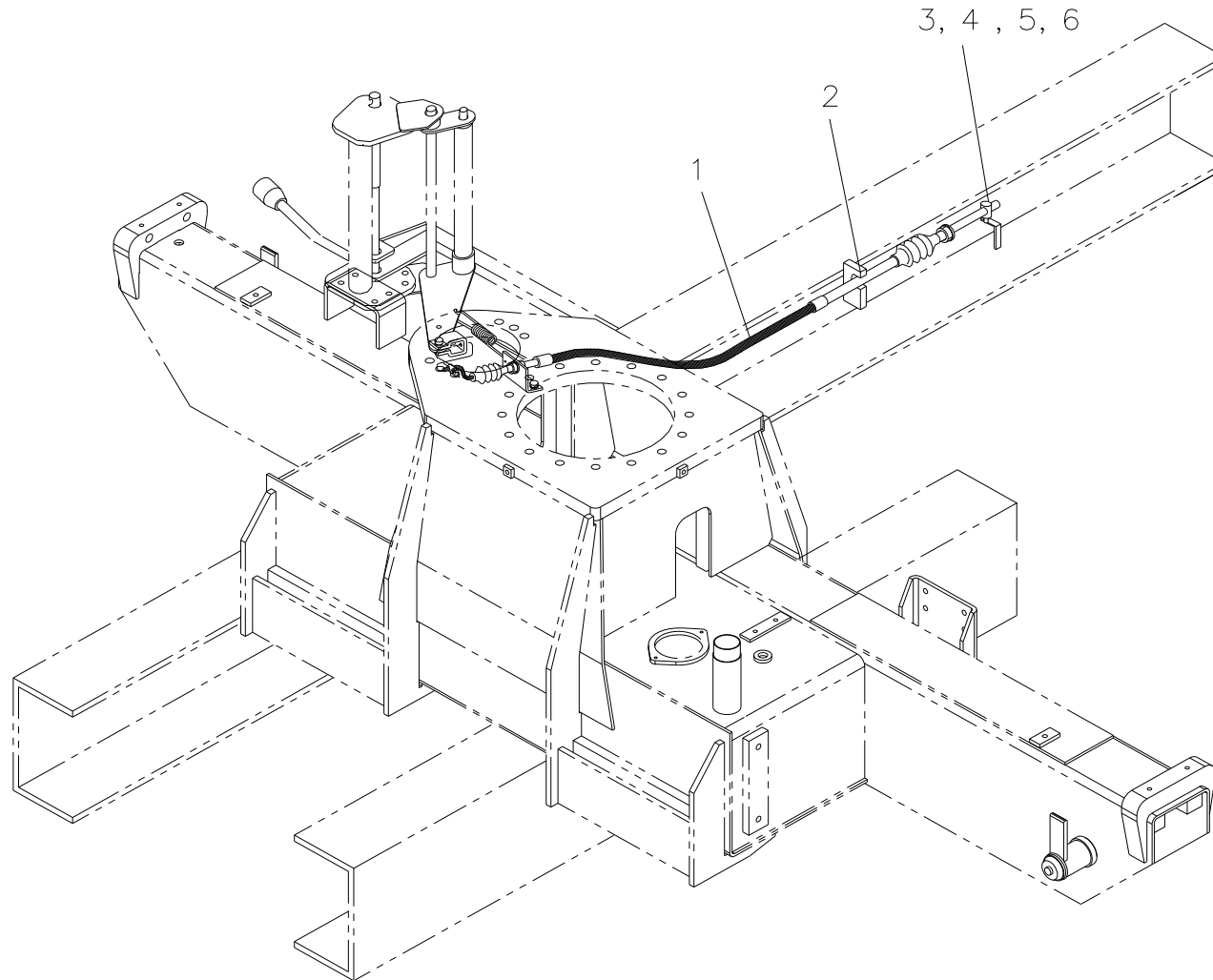
악셀 시스템 파트 Fig. 8-3 SAC-2501 ACC' SYSTEM PART
