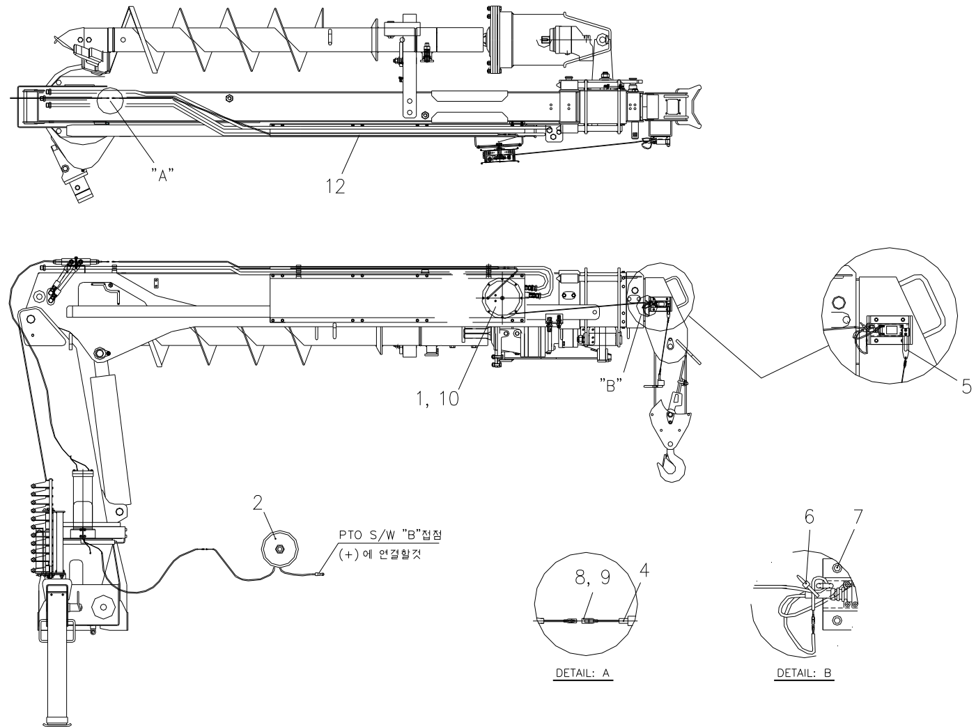
Fig. 11-1 SAC-2501 과권경보장치
