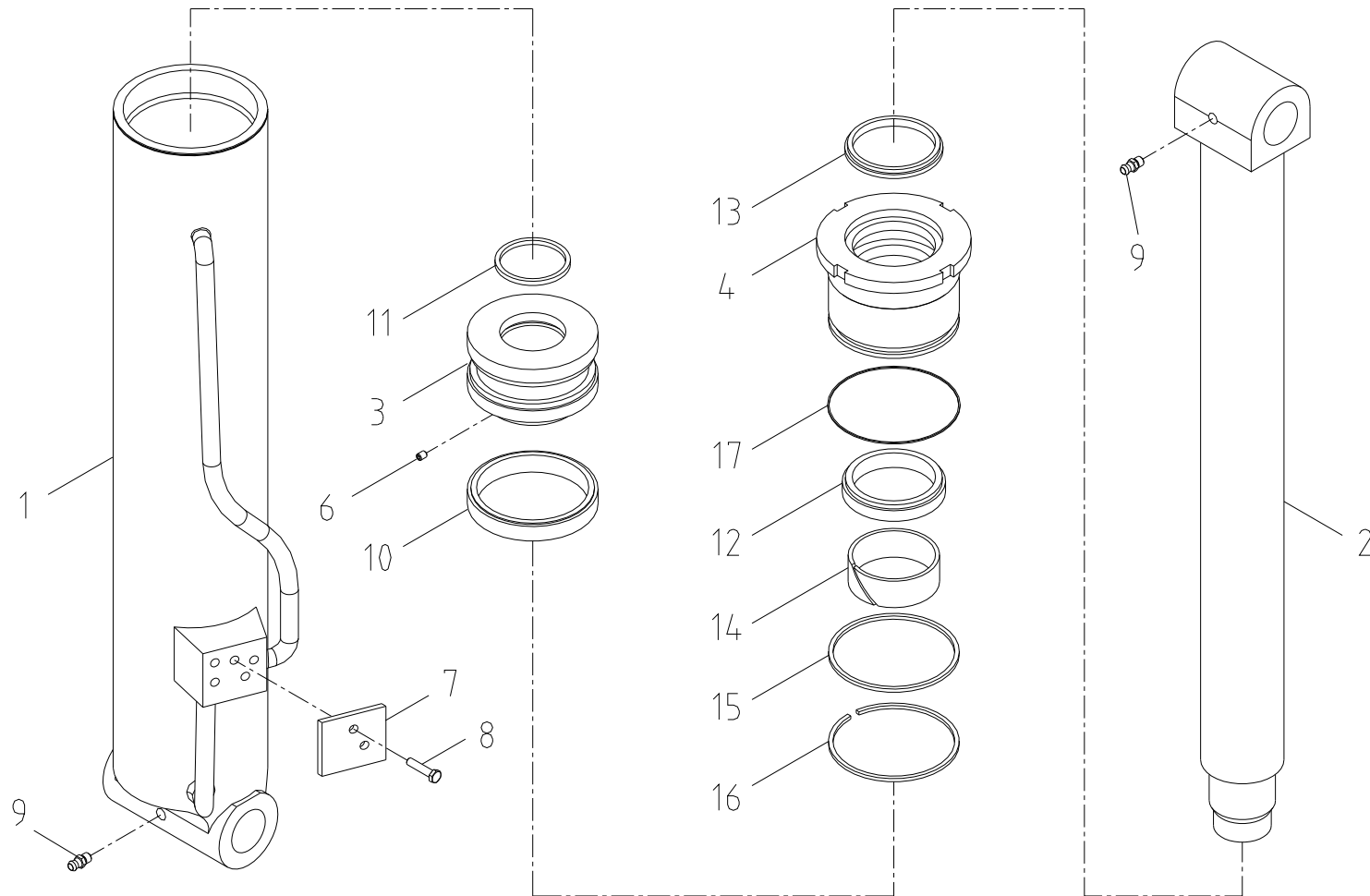
데릭 실린더 조립체 Fig. 2-2-1 SAC-2501 DERRICK CYL'D ASS'Y
