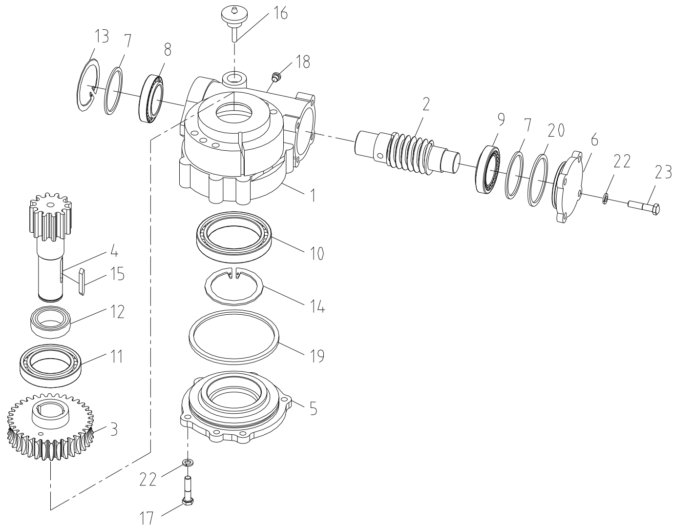
스윙 감속기 조립체 Fig. 2-1-2 SAC-2501 SWING R/G ASS'Y
