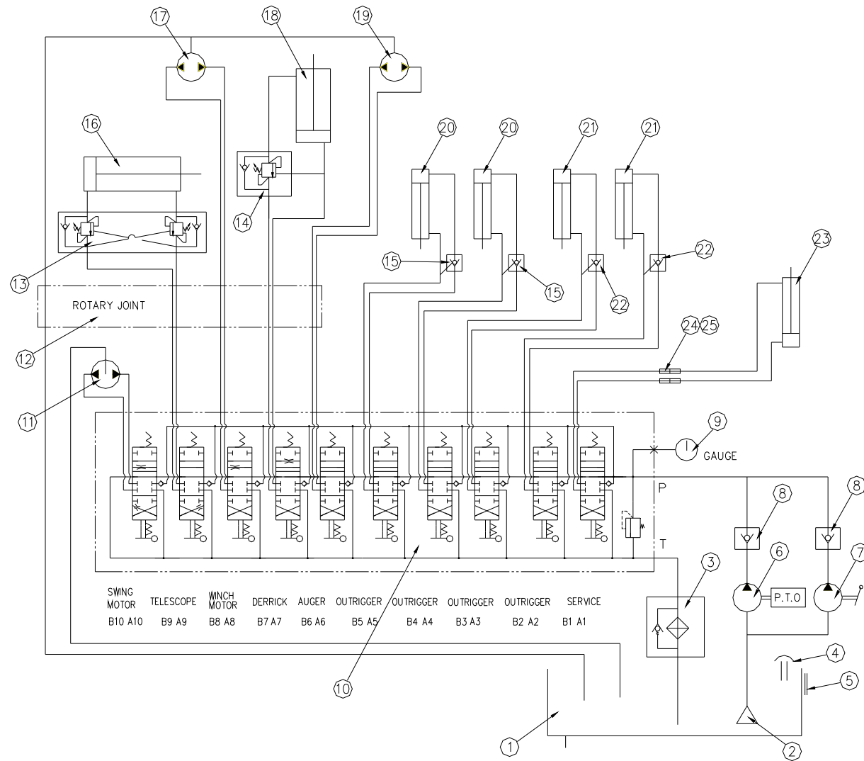
유압도 Fig. 10 SAC-2501 HYDRAULIC DIAGRAM
