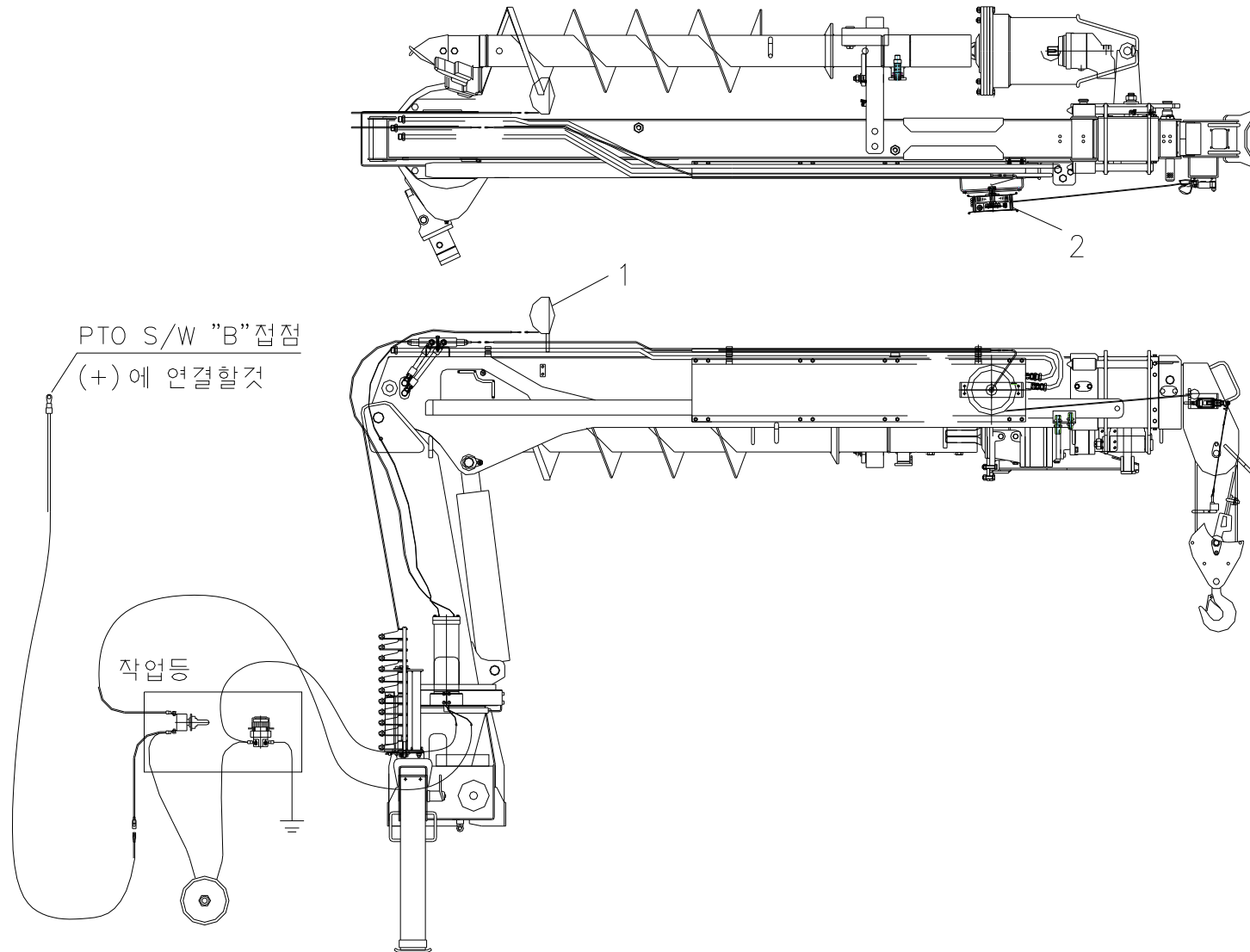
Fig. 11 SAC-2501 전기장치
