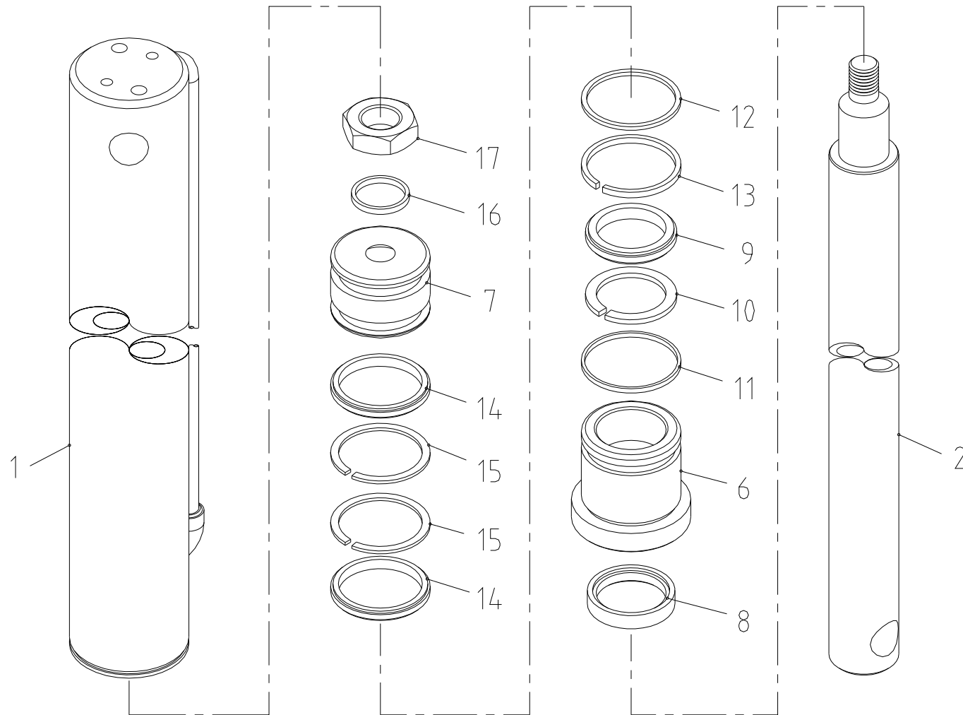
잭 실린더 조립체 Fig. 3-1 SAC-2501 JACK CYL' ASS'Y
